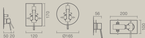
DUCHE / BANHEIRA 4 vias
