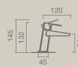
BIDÉ cascata fechada
