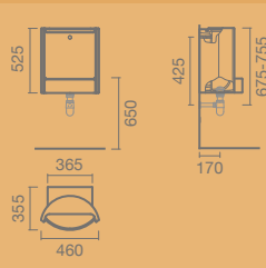
Entrada de água HORIZONTAL
