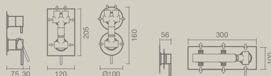
DUCHE / BANHEIRA 6 vias
