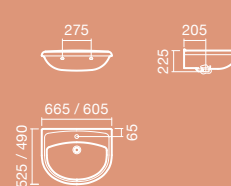
LAVATÓRIO 66 e 60
