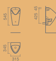
Entrada de água HORIZONTAL
