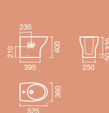
BIDÉ BTW
