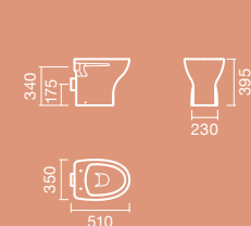
SANITA simples D/P
