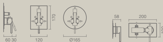
DUCHE / BANHEIRA 4 vias
