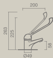
LAVATÓRIO manípulo clínico
