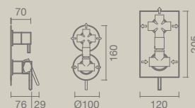
DUCHE / BANHEIRA 5 vias
