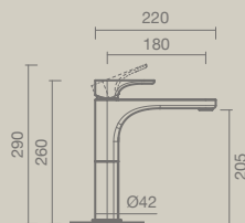
LAVATÓRIO cano alto
