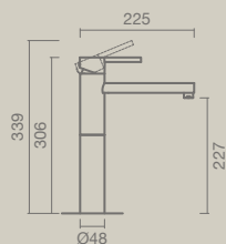
LAVATÓRIO cano alto
