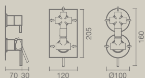
DUCHE / BANHEIRA 5 vias
