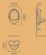
Entrada de água VERTICAL
