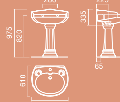
LAVATÓRIO 70
