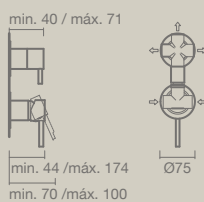
DUCHE / BANHEIRA 5 vias
