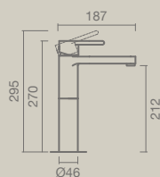
LAVATÓRIO cano alto
