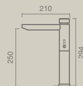
LAVATÓRIO cano alto: temporizada
