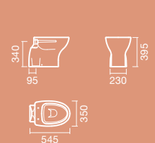
SANITA simples D/C
