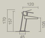
LAVATÓRIO cascata fechada
