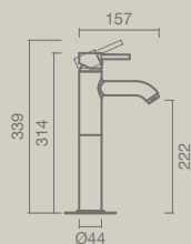
LAVATÓRIO cano alto
