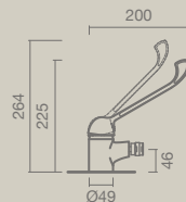
BIDÉ manípulo clínico
