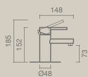
LAVATÓRIO
