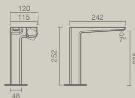
LAVATÓRIO cano alto
