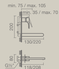
LAVATÓRIO de encastre
