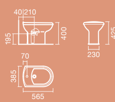
BIDÉ simples
