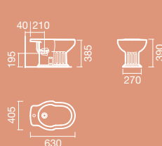
BIDÉ simples
